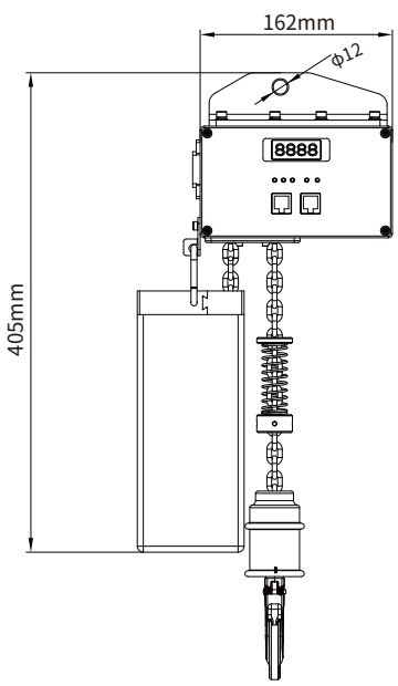
正视图
