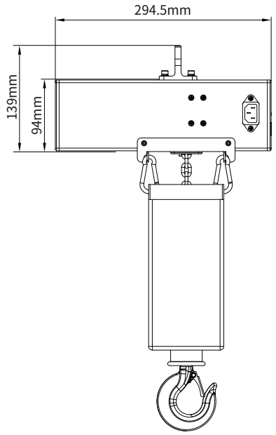
侧视图
