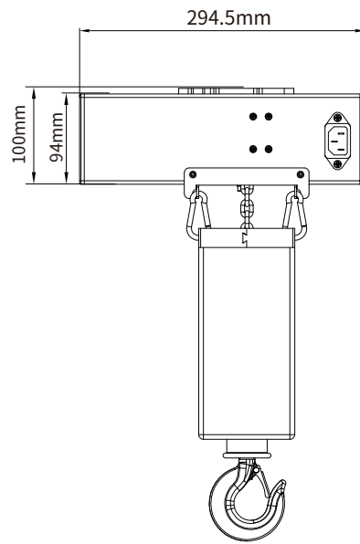
侧视图
