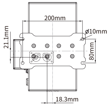
俯视图
