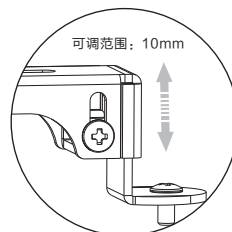
图十四 可调范围: 10mm
