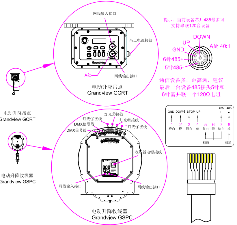
电动升降吊点、电动升降收线器接线详图
